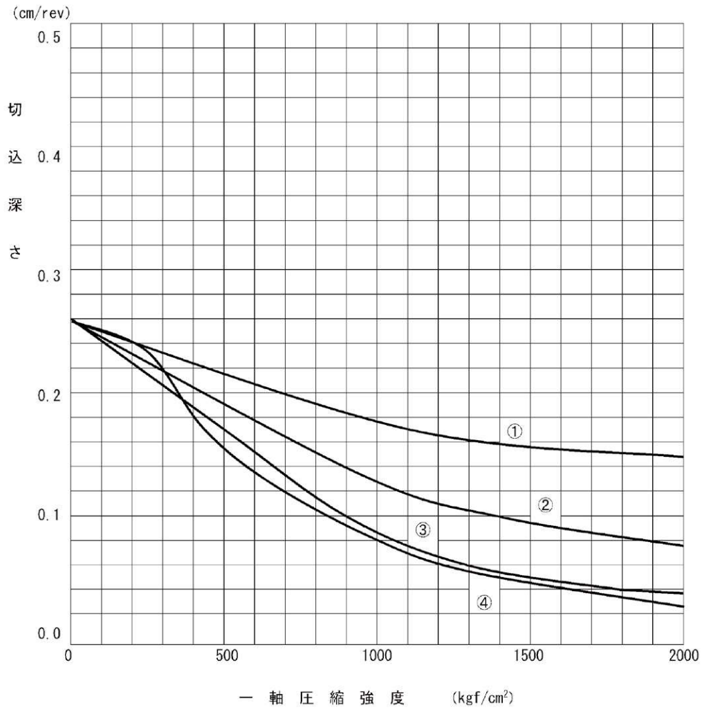
圧縮強度と切り込み深さ
