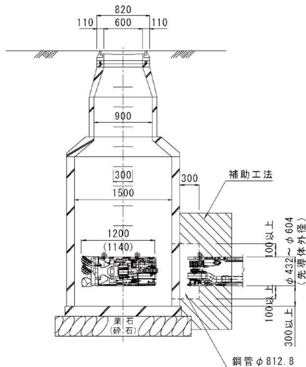
A-A 断面図
